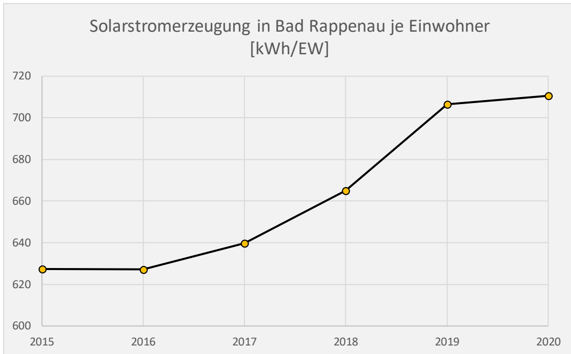
Abbildung 25: Jährlich erzeugter PV-Strom in Bad Rappenau mit Relation zur Einwohnerzahl
